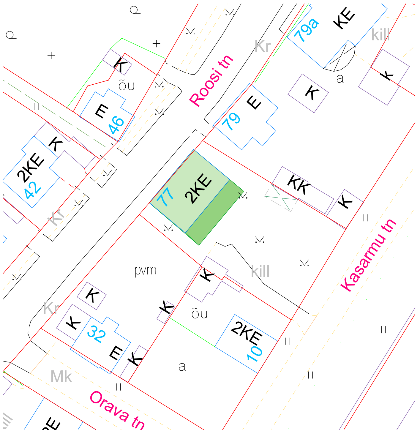
Lisa. Ehitusala skeem. Roosi tn 77 PTH-17-068
